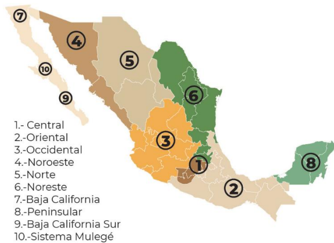
Ilustración 2. Regiones del Sistema Eléctrico Nacional
